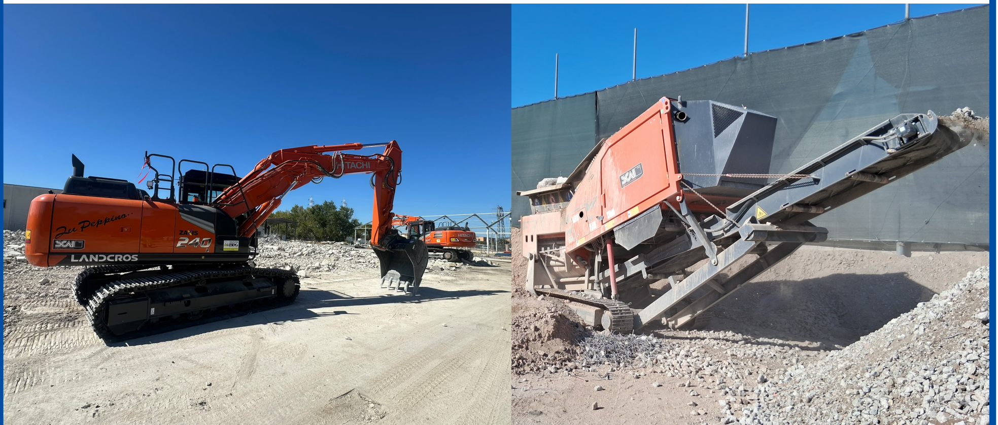
ESCAVATORE HITACHI ZX240NT-7 | TRITURATORE ARJES COMPAKTOR 300
